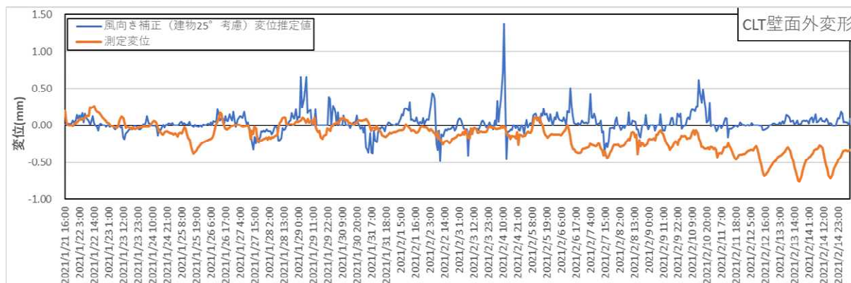
図 4.2.1 風圧力による外壁 CLT パネルの変形（風向き補正した変位と測定変位） （2021 年 1 月 21 日～3 月 31 日）
