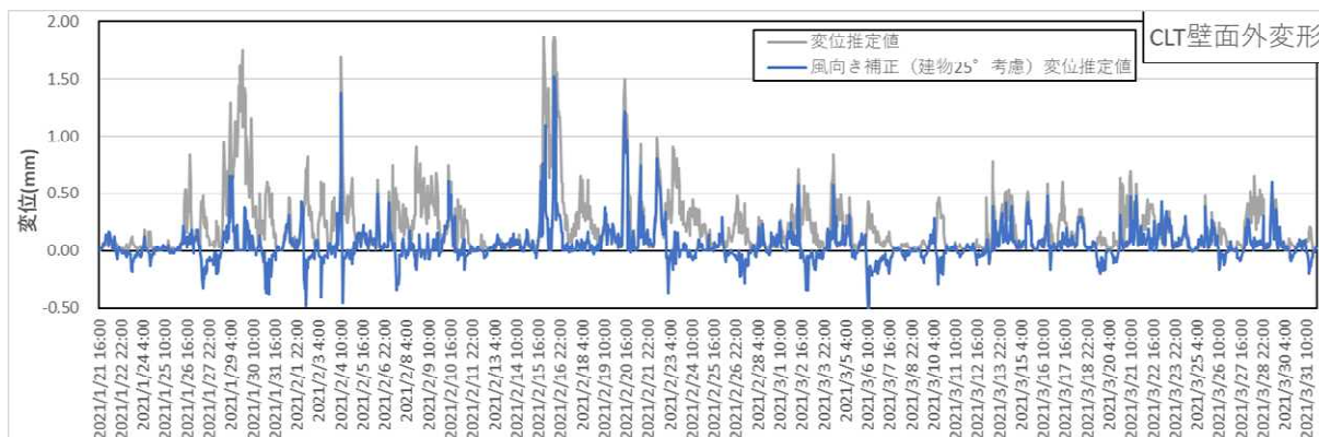
図 4.1.1 風圧力による外壁 CLT パネルの変形（風向き補正前による変位と風向き補正後の変位） （2021 年 1 月 21 日～3 月 31 日）
